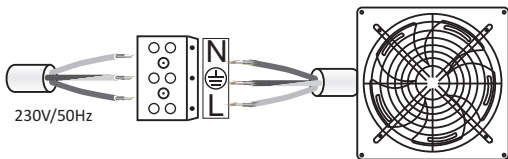
FIG. 2 - Wiring diagram
